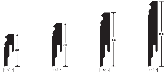
Fußleiste Profil 10 PK Fußleiste Profil 11 PK Fußleiste Profil 12 PK Fußleiste Profil 13 PK
