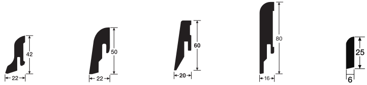
Fußleiste Profil 1 MK Fußleiste Profil 2 PK Fußleiste Profil 3 PK Fußleiste Profil 5 PK Fußleiste Profil 6
