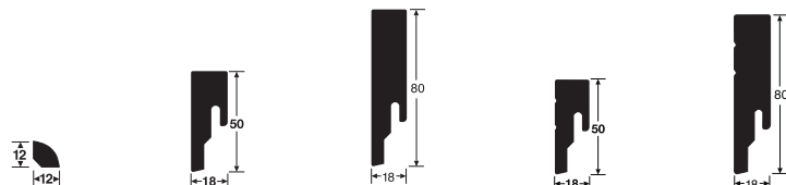
Viertelstab Profil 7 Fußleiste Profil 8 PK Fußleiste Profil 9 PK Fußleiste Profil 18 PK Fußleiste Profil 19 PK
