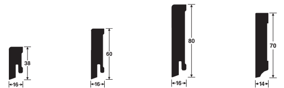
Fußleiste Profil 14 MK Fußleiste Profil 15 MK Fußleiste Profil 16 MK Fußleiste Profil 17
